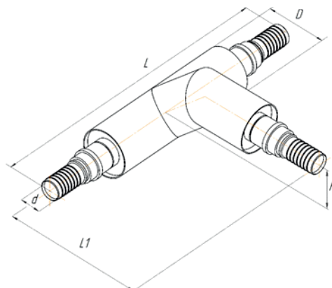
ГПИ тройник обжимной угловой равнопроходной
