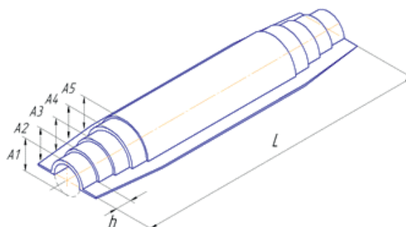
Кожух полимерный для изоляции пресс-муфты 225/160
